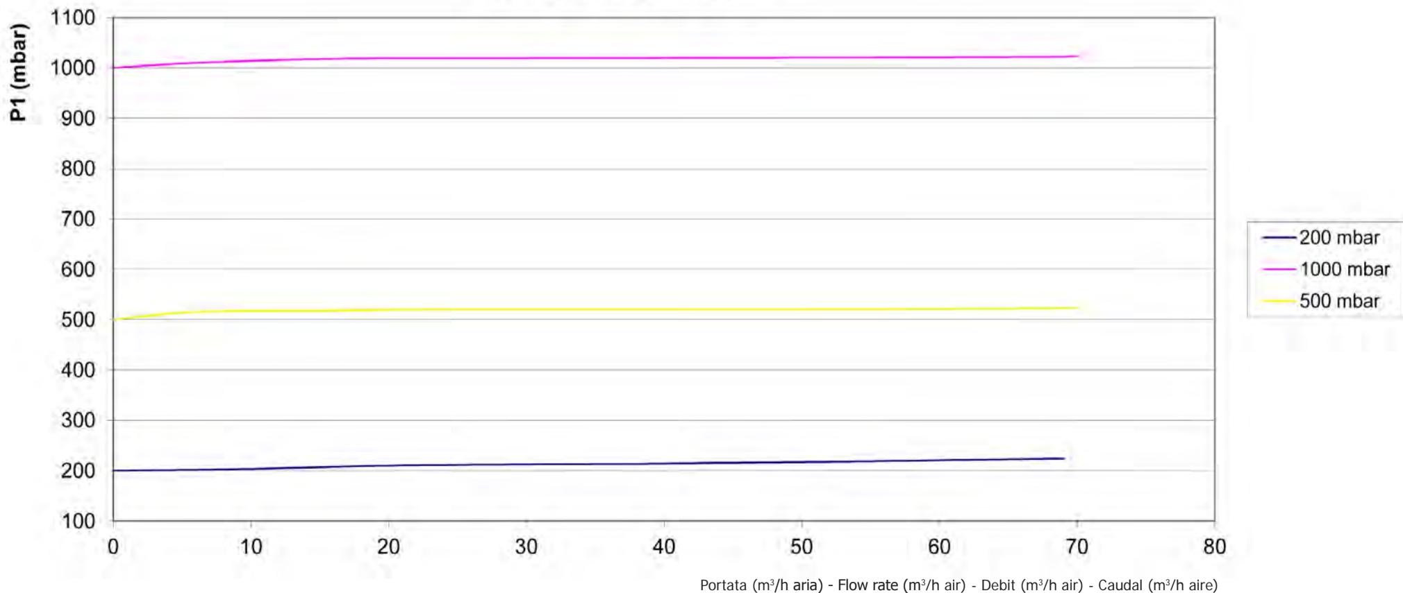
Range 200÷1000 mbar
