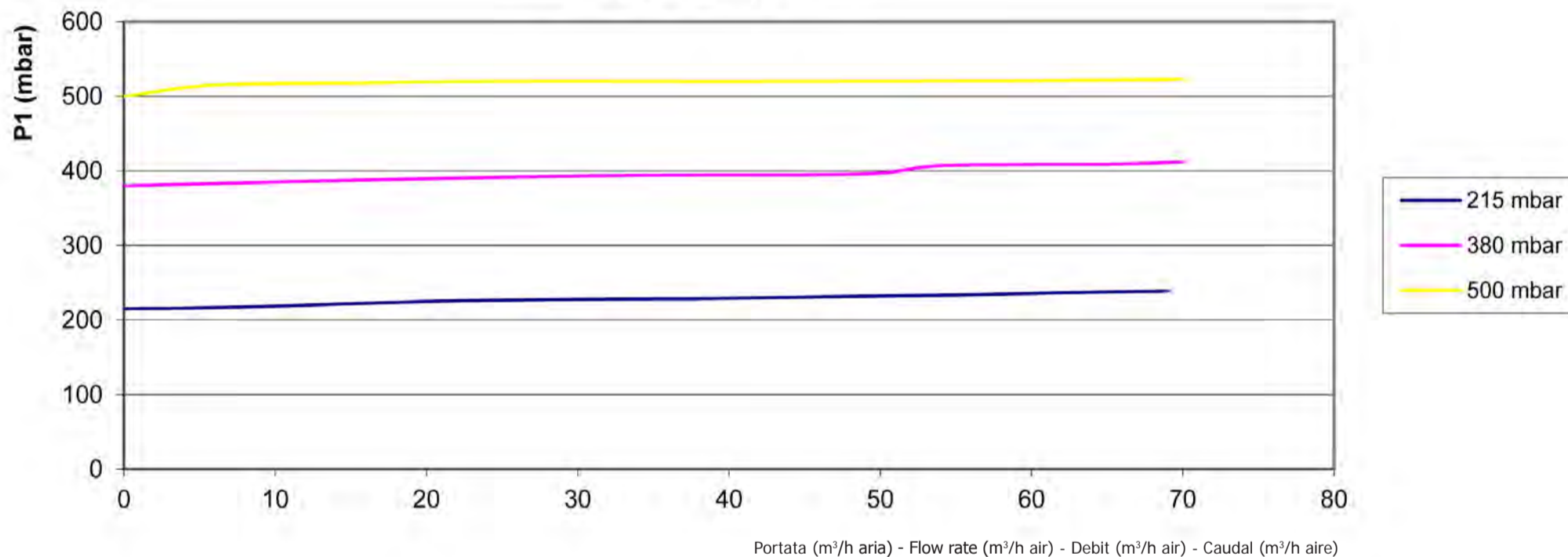
Range 215÷500 mbar
