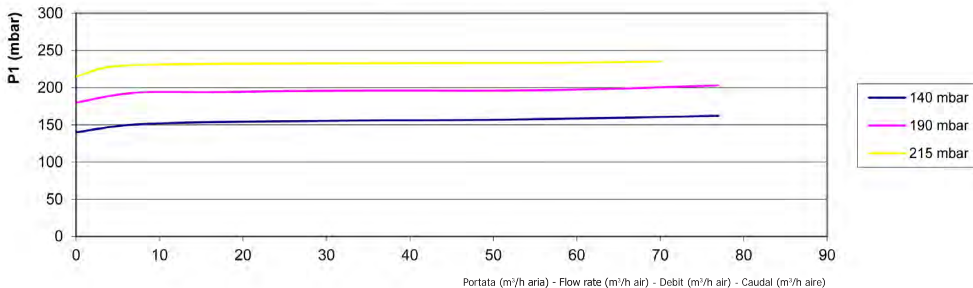
Range 140÷215 mbar
